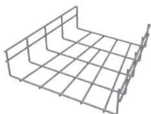
REDUÇÃO CONCÊNTRICA PLX - 310
